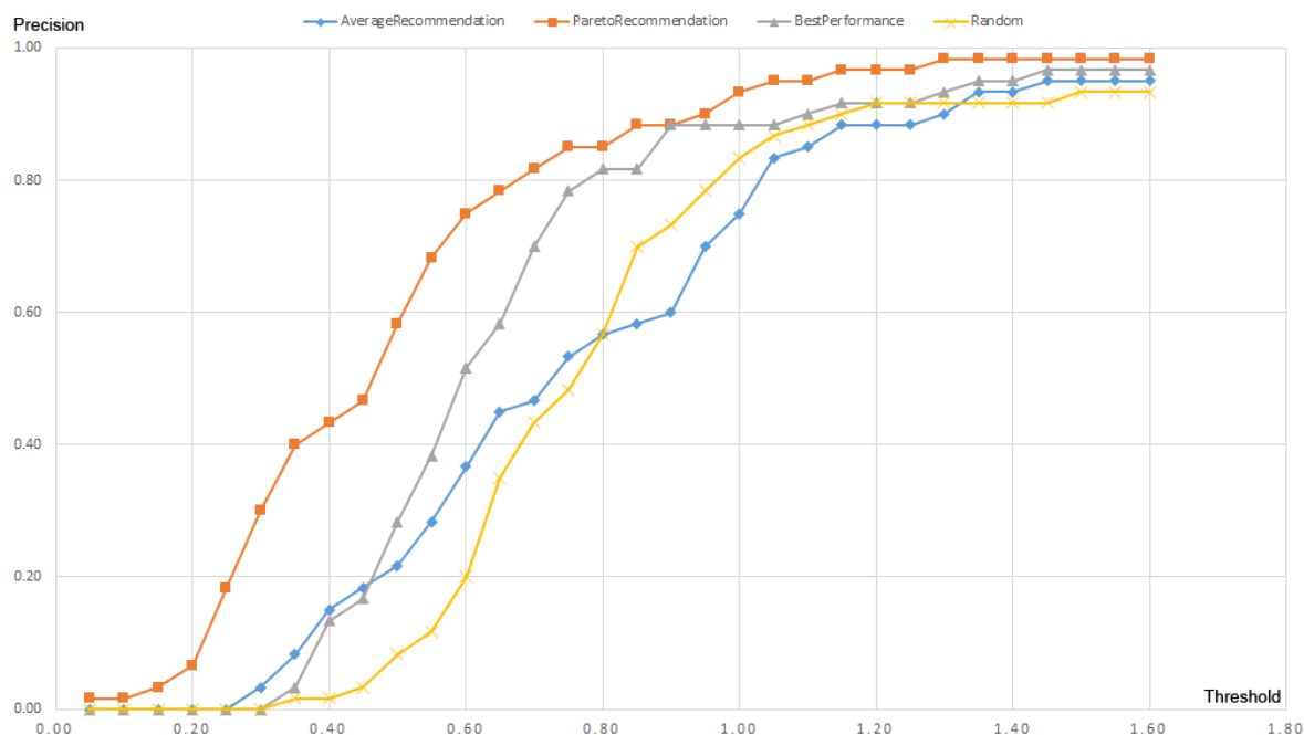
FIGURE 3.2 – Scores de précision par seuil de similarité, sur l'ensemble complet.
