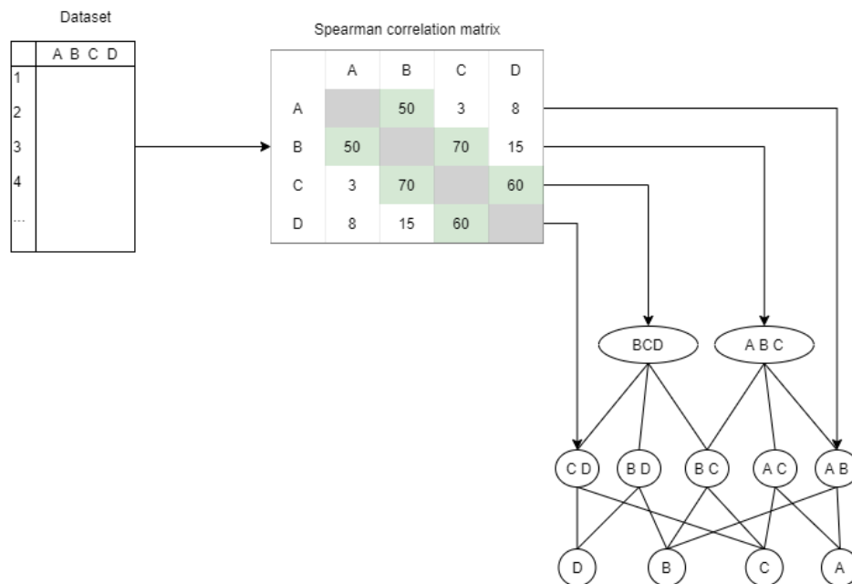
FIGURE 5.3 – Représentation des groupes calculés par la méthode de coalition basée sur la méthode de Spearman pour un jeu de données à 4 variables. La matrice de corrélation de Spearman est calculée. Pour chaque ligne, les variables les plus corrélées avec la variable courante de la ligne sont considérées comme faisant partie d'un groupe.
