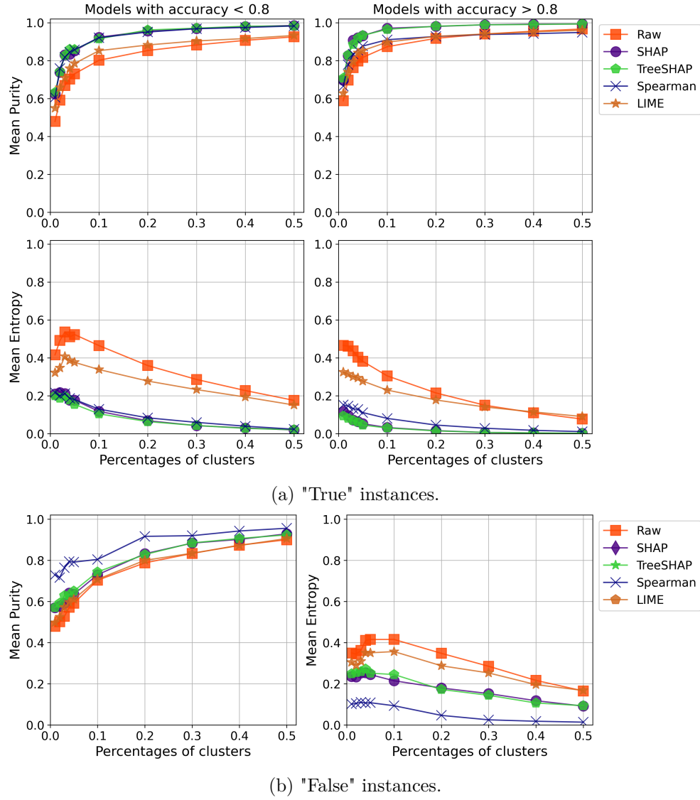
FIGURE 6.11 – Comparaison du clustering pour les méthodes XAI formées à partir (a) uniquement les "vraies" instances et (b) uniquement les "fausses" instances pour les modèles dont l'accuracy est inférieure à 0,8
