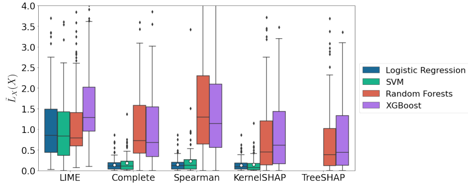
FIGURE 5.8 – Estimation locale de Lipschitz pour chaque modèle, regroupée par méthode. Chaque boîte représente les résultats agrégés pour tous les jeux de données. Le point blanc représente la valeur moyenne. En raison de valeurs aberrantes, nous avons repositionné le graphique à \tilde{L}_X(X) = 4
