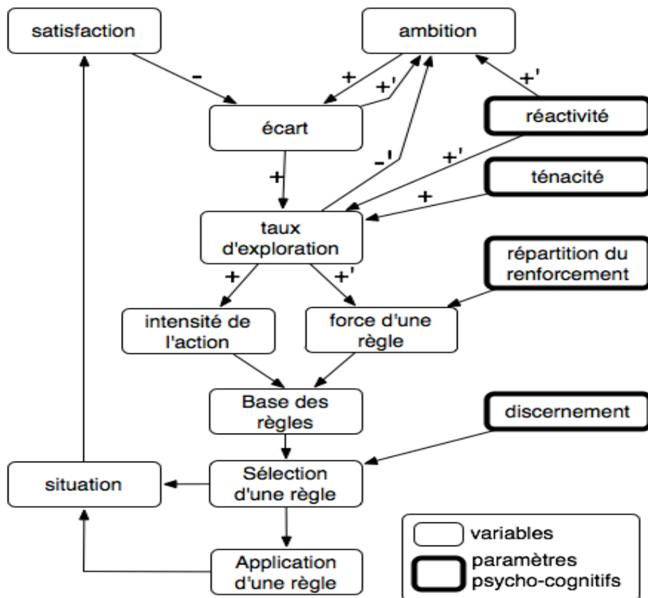
Figure 4.2. Relations de dépendance entre les variables et les paramètres de l'algorithme. Les arcs étiquetés "+" (resp. "-") indiquent une variation de même sens (resp. sens contraire) ; ceux étiquetés "+'" ou "-'" indiquent une influence sur le taux de variation, la dérivée, de la cible.
