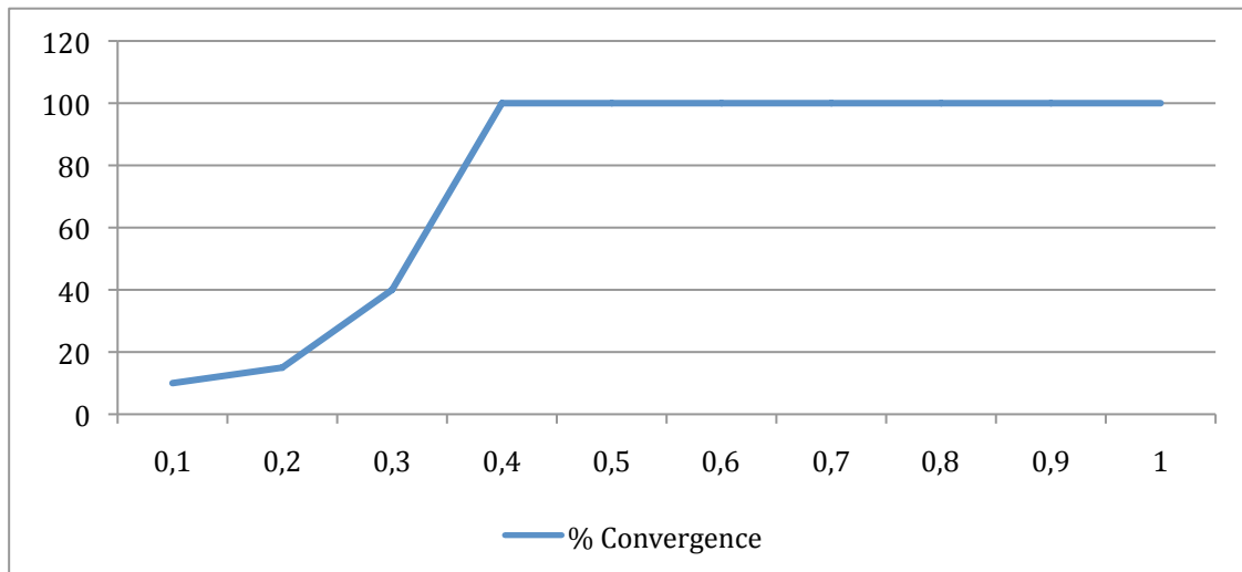
Figure 5.24. Le pourcentage de convergence des simulations en moins de 300 000 pas en fonction de l'égocentrisme des acteurs A2, A3, et A4 dans le modèle free-rider.
