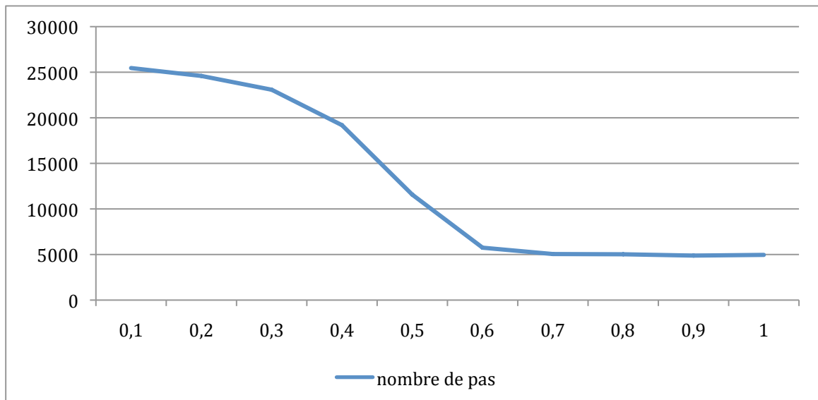
Figure 5.28. Le nombre de pas moyen pour les simulations, en fonction de l'égoïsme de A2 (A1 et A3 utilisent l'algorithme principal, tandis que A2 est égalitariste).
