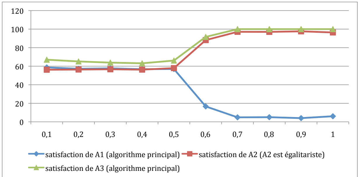
Figure 5.27. La moyenne de la satisfaction de chaque acteur en fonction de l'égoïsme de A2 (A1 et A3 utilisent l'algorithme principal, tandis que A2 est égalitariste).
