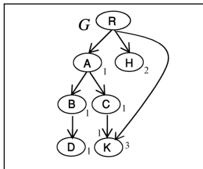
Figure III.5 - Exemple de structure de documents en graphe
