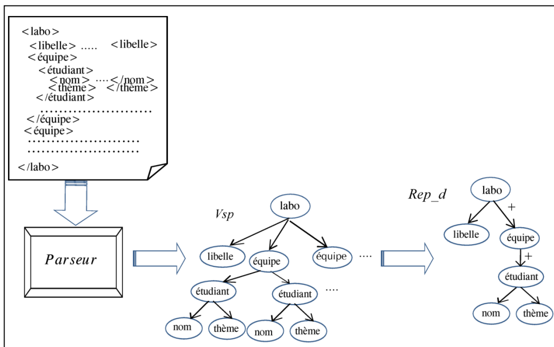
Figure III.15 - Chaîne d'extraction de la vue spécifique au représentant d'un document
