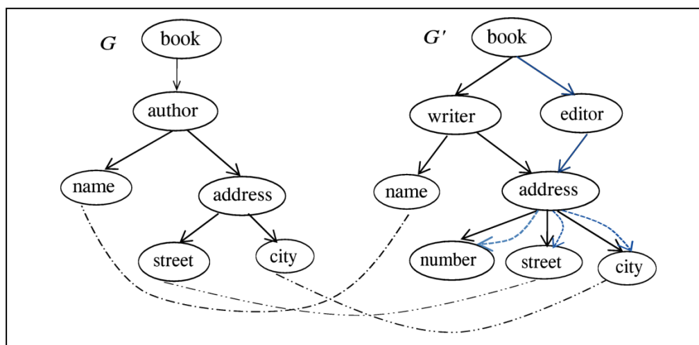
Figure III.7 - Exemple d'appariement de chemins : étiquettes synonymes
