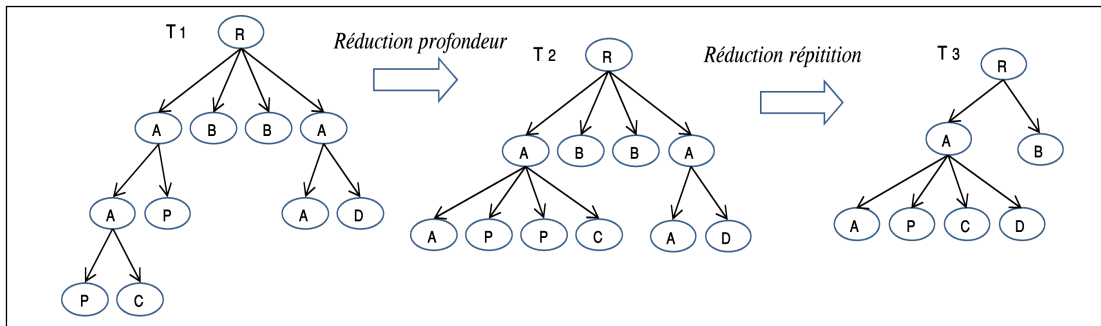
Figure II.16 - Extraction du résumé structurel [Dalamagas T. et al., 2006]
