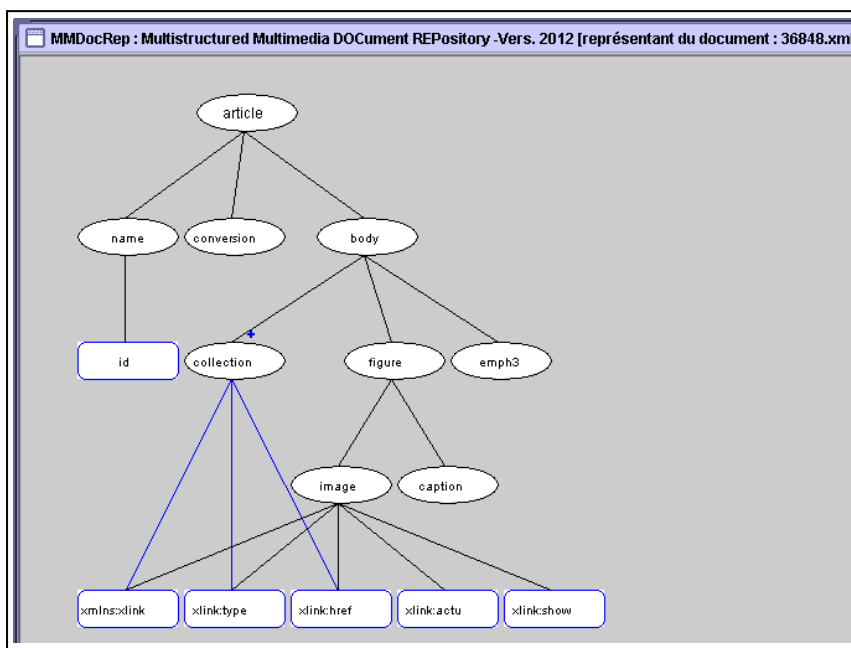
Figure III.18 - Exemple de représentant Rep_d du document de la figure 16
