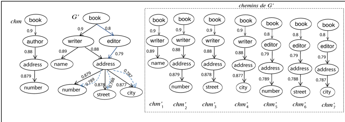
Figure III.8 - Exemple d'inclusion d'un chemin dans un graphe
