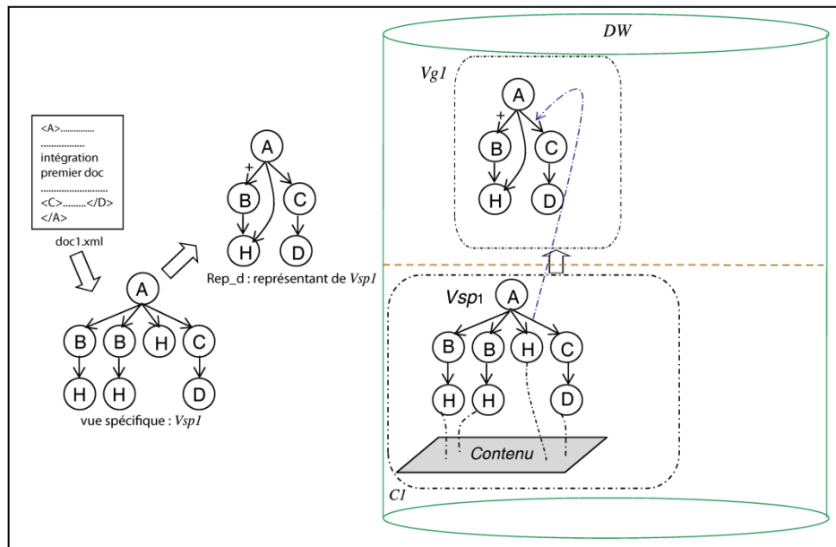
Figure 6 : Intégration du premier document
