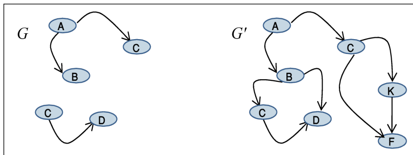
Figure II.7 - Sous-graphe partiel d'un graphe
