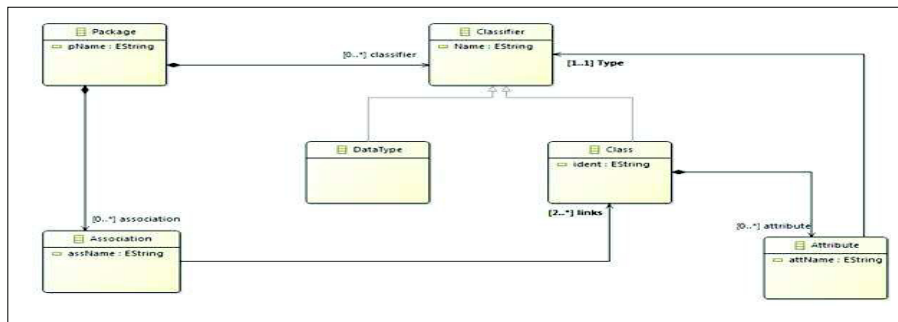
Figure 3. Méta-modèle source
