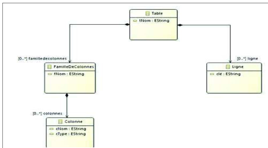
Figure 4. Méta-modèle cible
